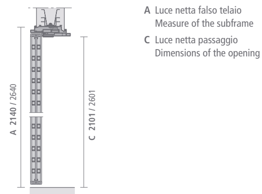
Slim Porta battente Swing door
